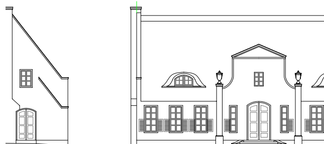
Ansicht Nord-Ost
